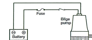
Zapojení pro manuální provoz
