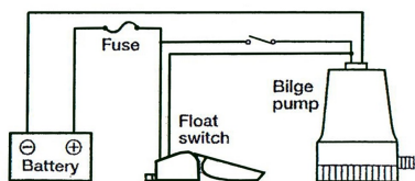
Zapojení pro automatický provoz
